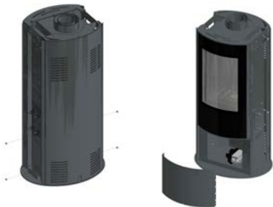
Fig. 9 Méthode de retirer la porte inférieure du chauffage Koza AB GAZ
