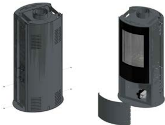
Rys. 9. Sposób demontażu drzwi dolnych w ogrzewaczu Koza AB GAZ
