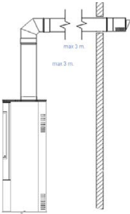
Rys. 5. Sposób wyprowadzenia koncentrycznego systemu kominowego
